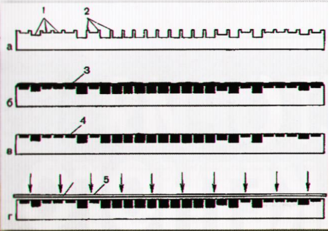
Рис. 3 Схема глубокой печати. 1, 2 – печатная форма в разрезе, показаны углубления, которые заполняются краской, и пробельные выступы; 3 – нанесённый слой краски; 4 – остатки краски в углублениях после прохода ракеля; 5 – бумага
