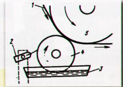
Рис. 7 Схема рапельной (растровой) глубокой печати. 1 – бумага; 2 – рапель; 3 – красочный резервуар; 4 – формный цилиндр; 5 – печатный цилиндр
